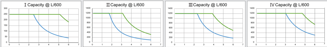
Y轴 = 负载+提升装置重量 (kg) X轴 = 悬挂距离 (m) 轨道承载力数据图
